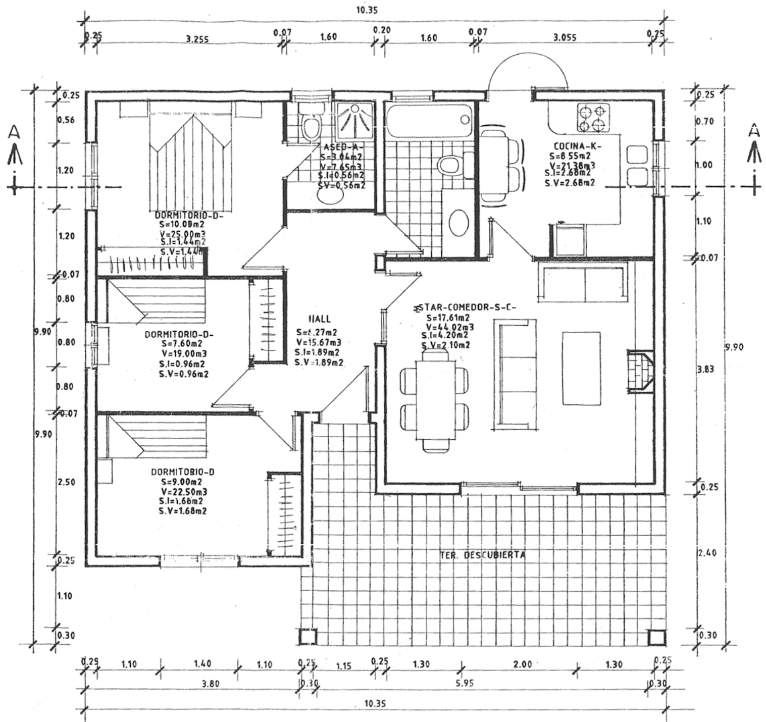
PLANTA BAJA
